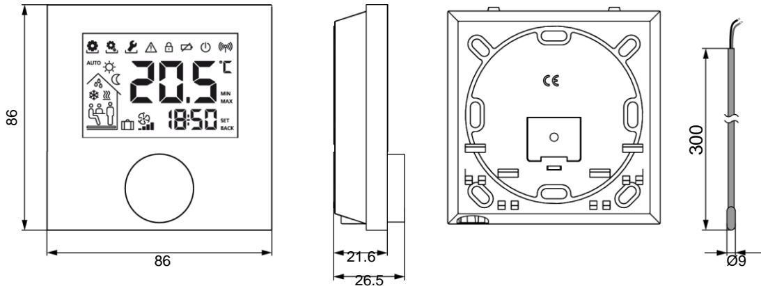
Figure 1: Dimensions OEM Alpha 2: Raumbediengeräte Funk mit Display and external sensor (indications in mm)
