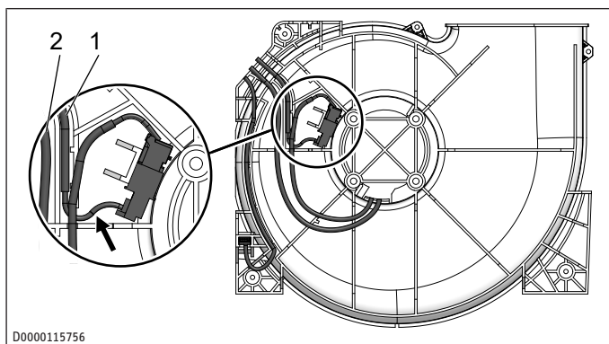
1 Omrežni kabel ventilatorja 2 Krmilni kabel ventilatorja
