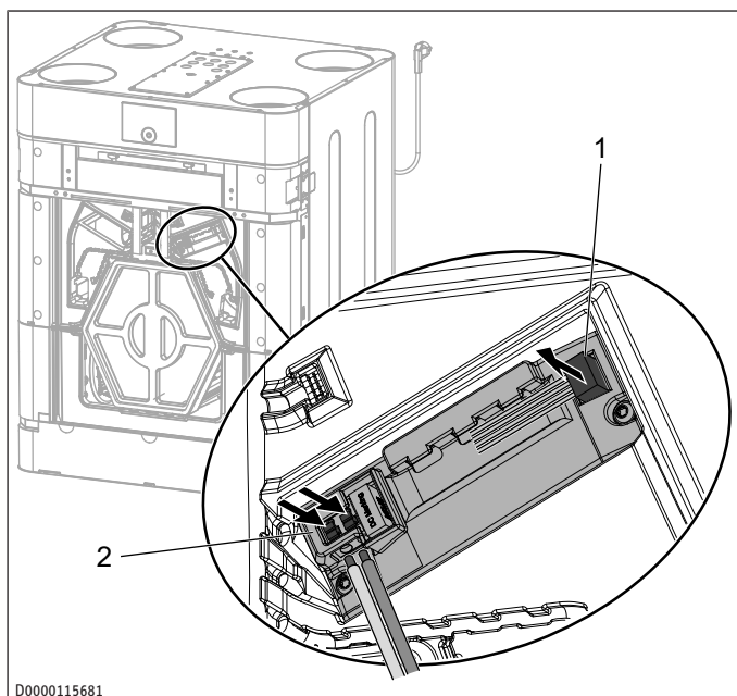
1 Circuit de commande
