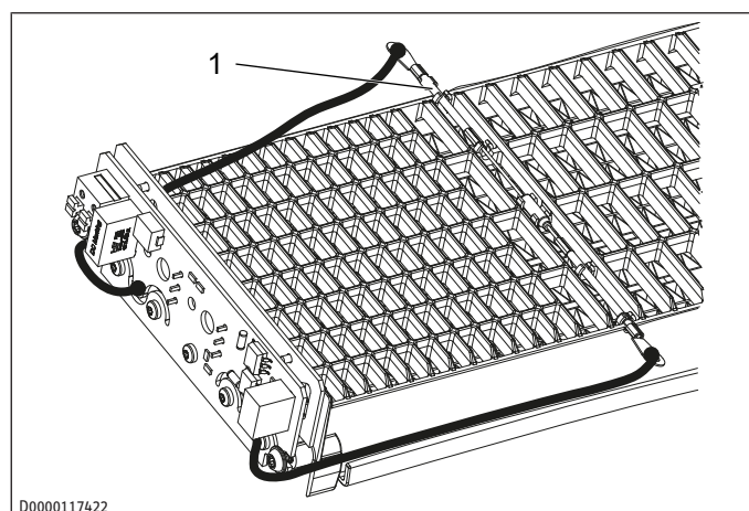
1 Bezpečnostní konstrukční skupina
