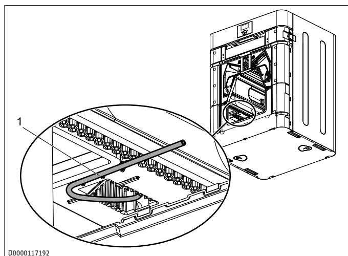
1 Support du tuyau antivibratoire
