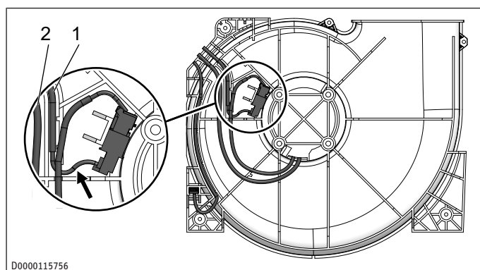
1 Câble d'alimentation du ventilateur 2 Câble de commande du ventilateur
