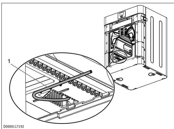
1 Supporto del tubo di misura della prevalenza
