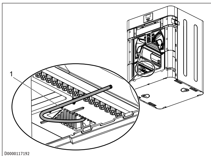
1 Držalo tlačne cevi
