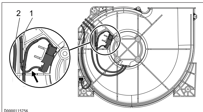
1 Cavo di alimentazione del ventilatore 2 Cavo di controllo del ventilatore
