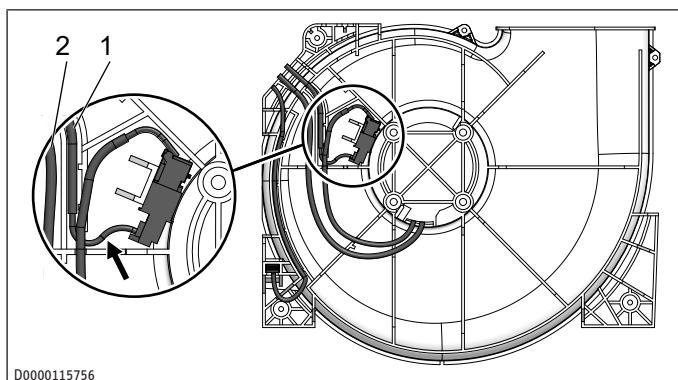
1 Napájecí kabel ventilátoru 2 Řídicí rozvod ventilátoru
